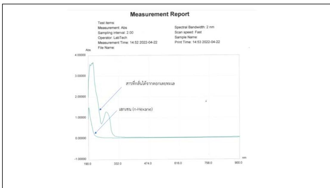
รูปที่ 18 สเปกตรัมการดูดกลืนแสงย่านวิชิเบิลของส่วนที่กลั่นได้ของดอกเตยทะเล
